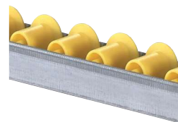
Válečkové lišty s válečky s nákolkem Ø 18/28 mm
