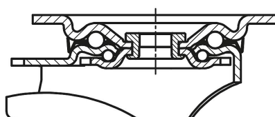
Uložení otočného věnce:
