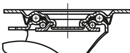
Uložení otočného věnce:
