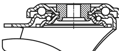
Uložení otočného věnce:
