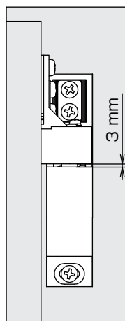
上ヒンジ Upper Hinge
