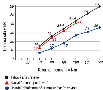
Diagram upínací síly 5osé upínače KIPPflexX
