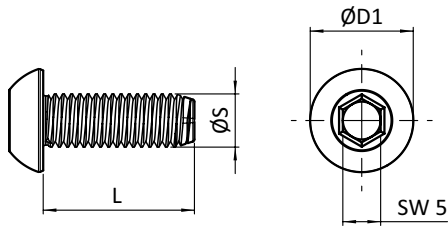
Selbstformende Halbrundschaube Self Forming Button Head Screw
