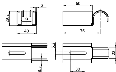
Variable Halter ST D28 Variable Holding Bracket ST D28
