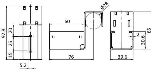
Einhängehalter ST D28 Holding Bracket ST D28
