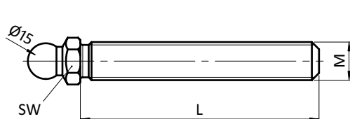
Gewindestange Stahl für Gelenkstellfüße, Kugel 15 Threaded Rod for Swivel Feet, Ball Joint 15
