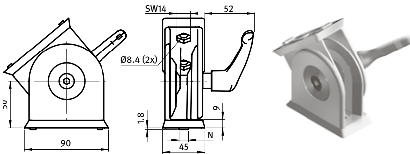
Gelenk 45 × 90 mit Klemmhebel Pivot Joint 45 × 90 with Locking Lever
