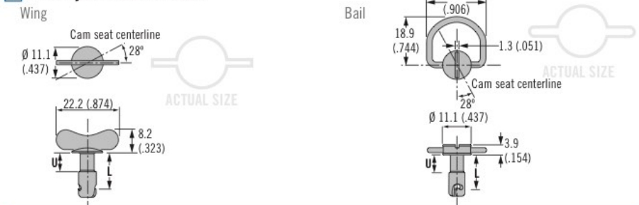
Stud Length Table
