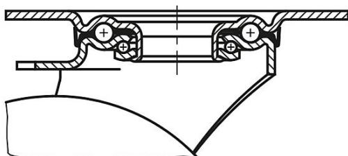
Uložení otočného věnce do R1 = 125
