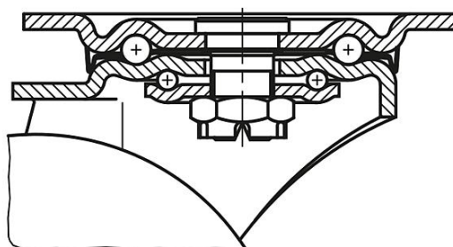
Uložení otočného věnce od R1 = 160
