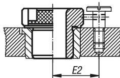
Rychlovýmenné pouzdro provedení K s vrtacím pouzdrům s nákrůžkem podle DIN 172 nebo s vrtacím pouzdrům podle DIN 179
