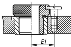
Výmenné pouzdro provedení L s vrtacím pouzdrům s nákrůžkem podle DIN 172 nebo s vrtacím pouzdrům podle DIN 179
