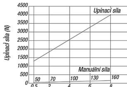
Přítlačný upínač 04565-0800 04565-0801
