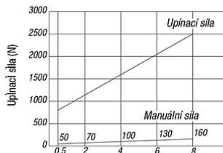
Tahový upínač 04400-4050...
