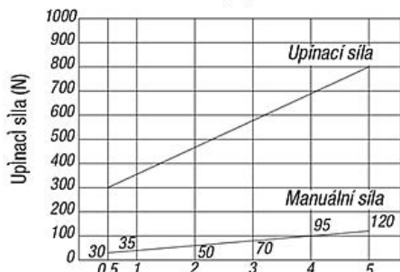
Otočný upínač 04366-...3232
