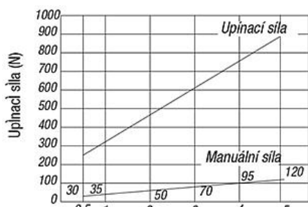
Tahový upínač 04400-3240...
