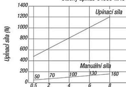
Otočný upínač 04366-...4540
