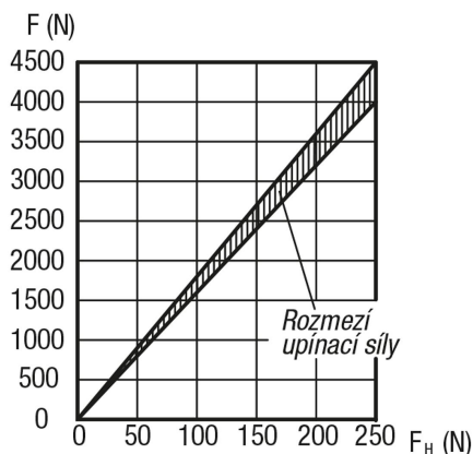
Silový diagram
