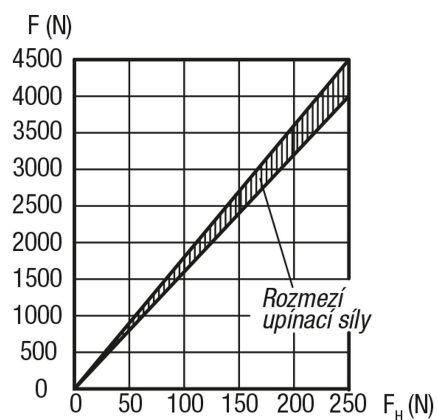
Silový diagram
