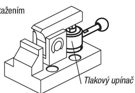
Vertikální upínání
