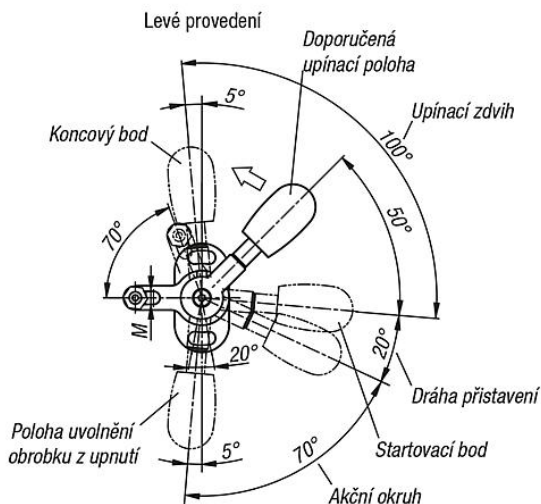
Levé provedení
