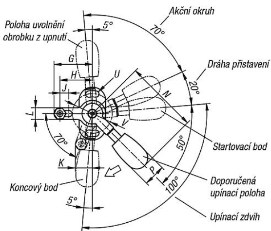
Pravé provedení
