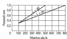
Posunutí při statickém zatížení z jedné strany
