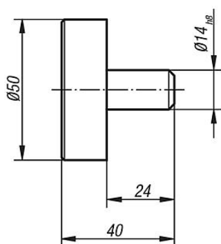
válec
