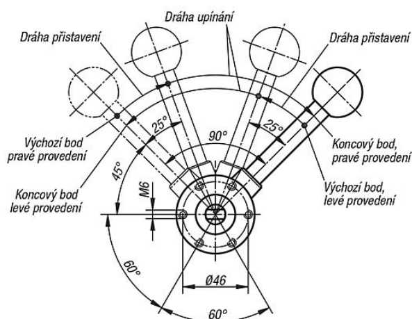
Pohled zdola
