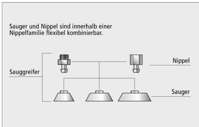
Baukastensystem Sauggreifer
