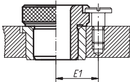
Auswechselbuchse Form L mit Bundbohrbuchse nach DIN 172 oder Bohrbuchse nach DIN 179
