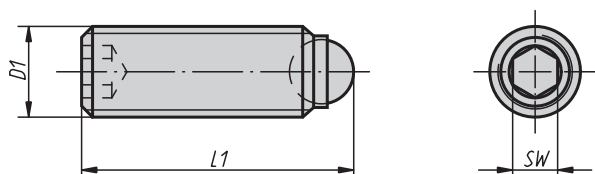
Provedení A s plnou kuličkou
