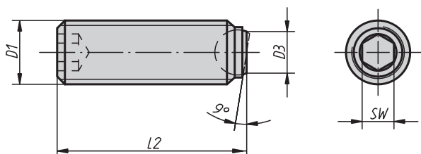
Provedení B se zploštělou kuličkou
