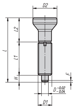
Aretační čep s klíčem
