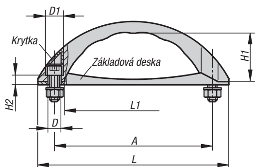
Provedení A se základovou deskou
