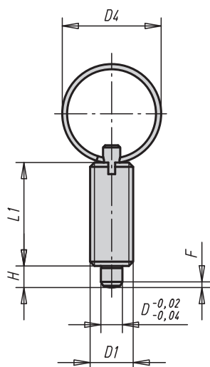
Provedení T bez protimatice
