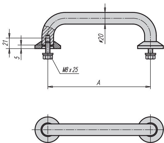
Provedení B k přišroubování na zadní stranu
