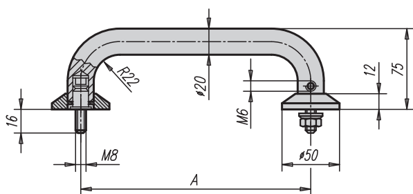
Provedení A k přišroubování na přední stranu
