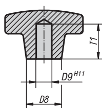
Provedení G slepý otvor
