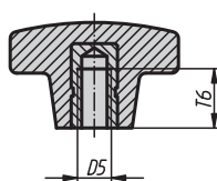
Provedení K s pouzdem se závitem
