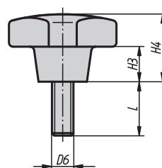
Provedení L s vnějším závitem
