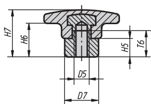
Provedení E s předsazeným ocelovým pouzdem
