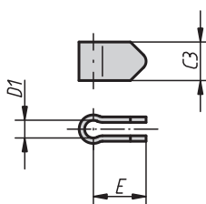
Objímka šroubu s možností přivaření
