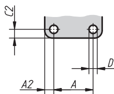
Děrová šablona pro obj.č. 05790-0450
