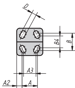
Děrová šablona pro obj.č. 05720-0200
