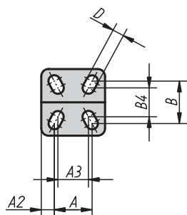
Děrová šablona pro obj.č. 05720-0100
