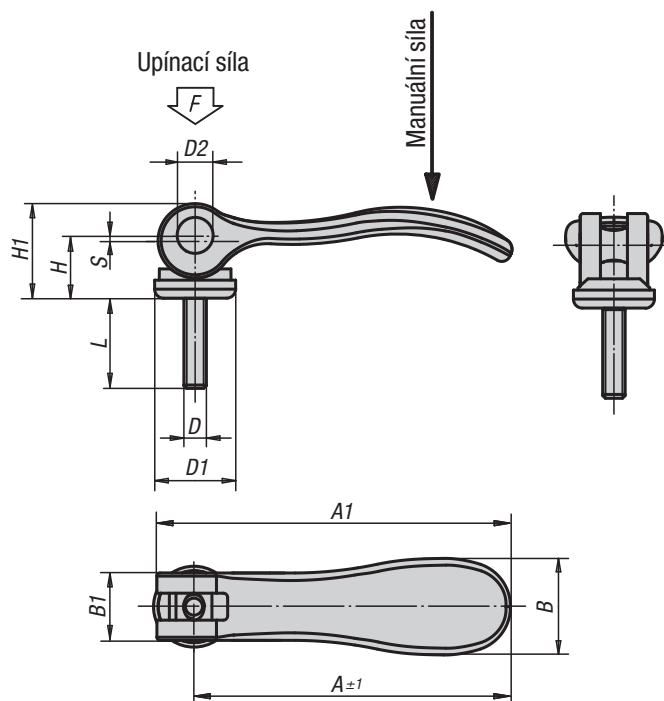
Excentrická páka s vnějším závitem
