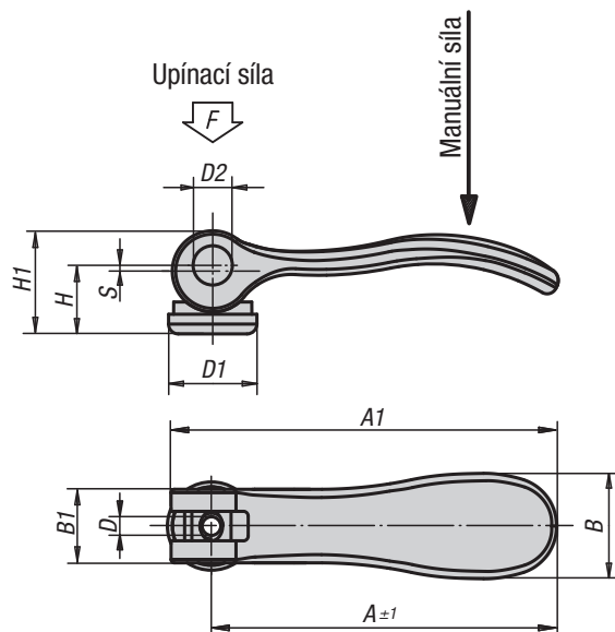
Excentrická páka s vnitřním závitem
