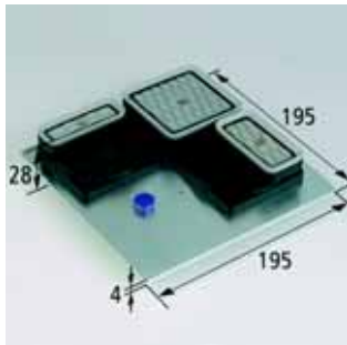
Ansiht von unten ISAP-S1
